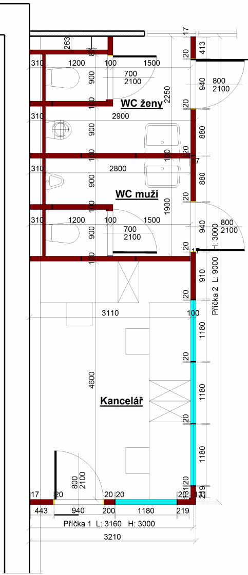
Příčka 1
