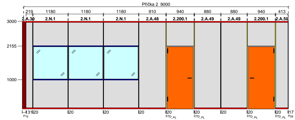
Příčka 2
