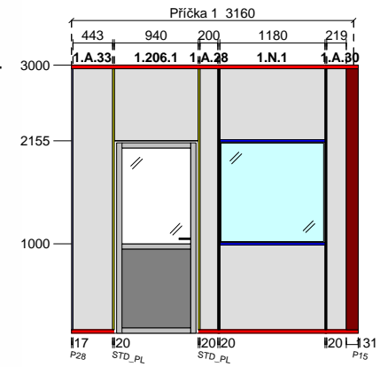
Příčka 1
